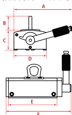
《ウルトラリフト TP のサイズ》
