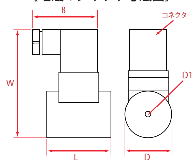
《電磁マグネット寸法図》
