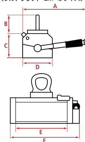
《ウルトラリフト LM のサイズ》
