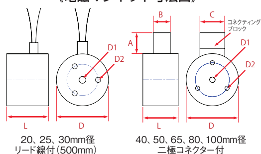
《電磁マグネット寸法図》
