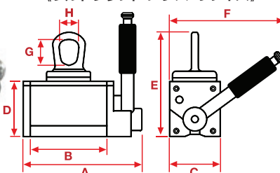
《ウルトラリフト プラスのサイズ》
