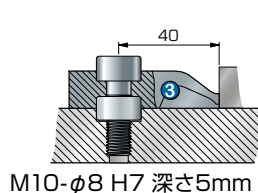
M10-φ8 H7 深さ5mm
